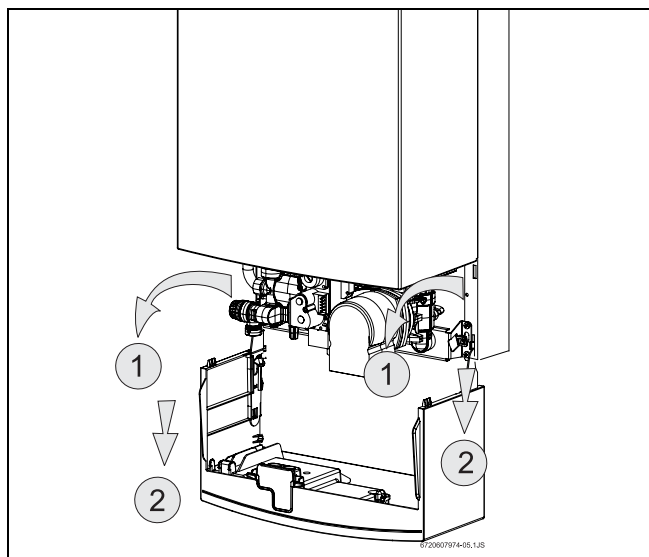
Рис 24 Сервисное положение для доступа к системам водо- и электроснабжения
