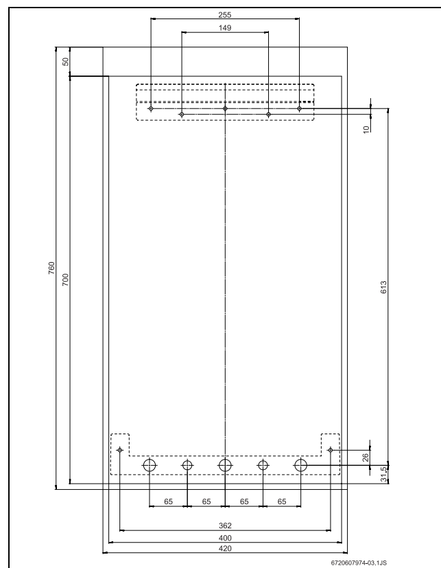
Рис 6 Комплект для настенного монтажа
