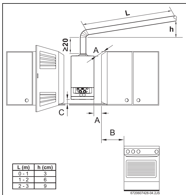
Рис 5 Минимальные расстояния
