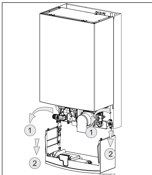
Рис 8 Сервисное положение для доступа к системам водо- и электроснабжения.
