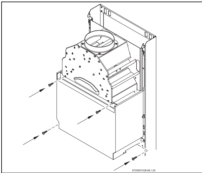
Рис 22 Защитная панель
