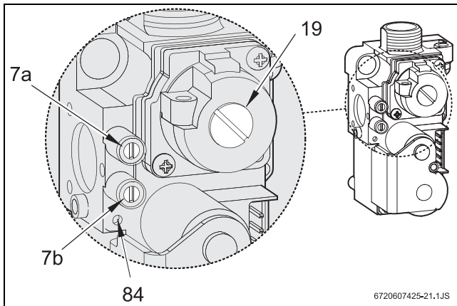
Рис 21 Газовая арматура
