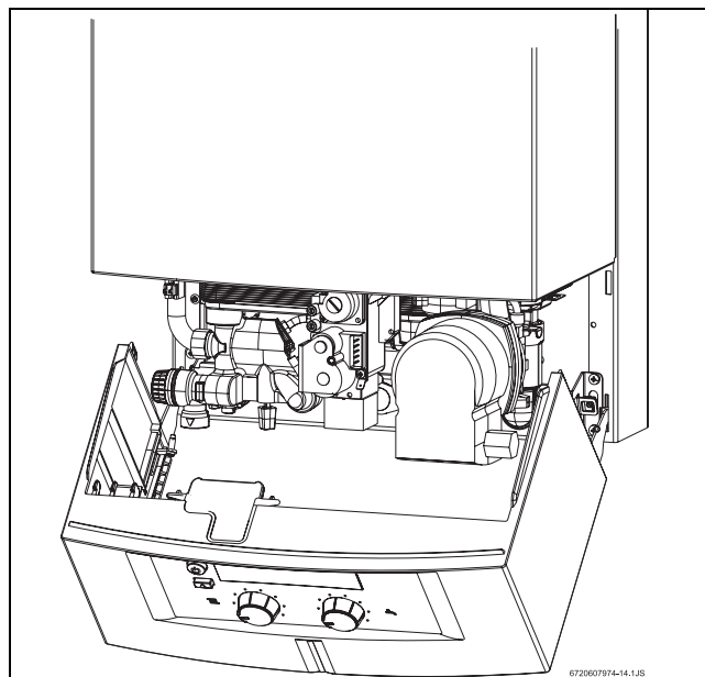
Рис 20 Сервисная позиция для регулирования газовой арматуры
