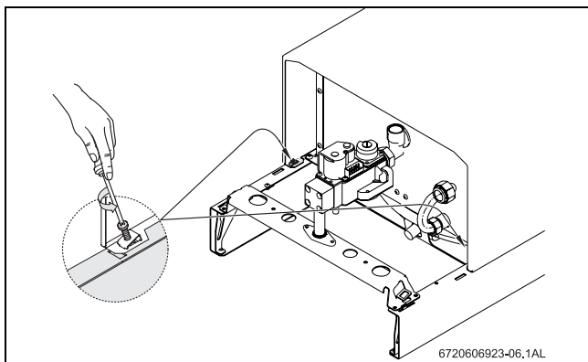
Рис 10 Снять переднюю крышку
