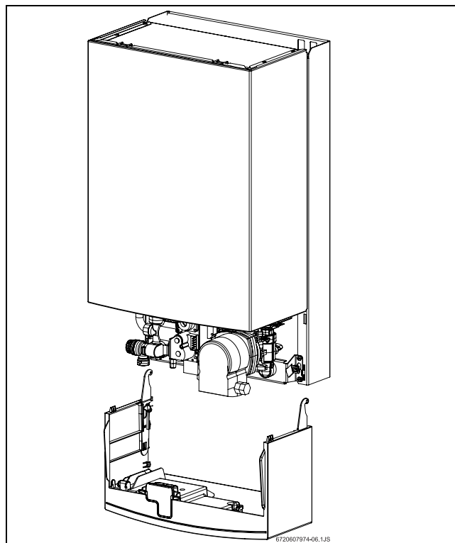
Рис 9 Съём коробки панели управления
